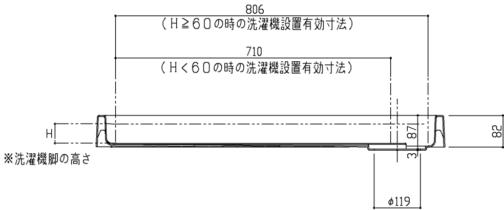
断面A-A
